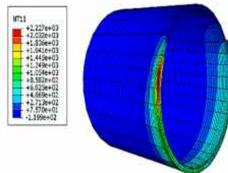
شکل ۲- توزیع دما حین فرایند جوشکاری
