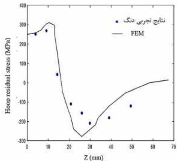
شکل ۱- مقایسه نتایج تجربی دنگ و مدل‌سازی المان محدود انجام شده
